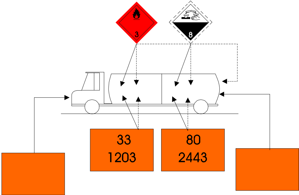
Fig. 5 Vehículo Cisterna cargados con dos o más Mercancías Peligosas de distinta Clase o División
