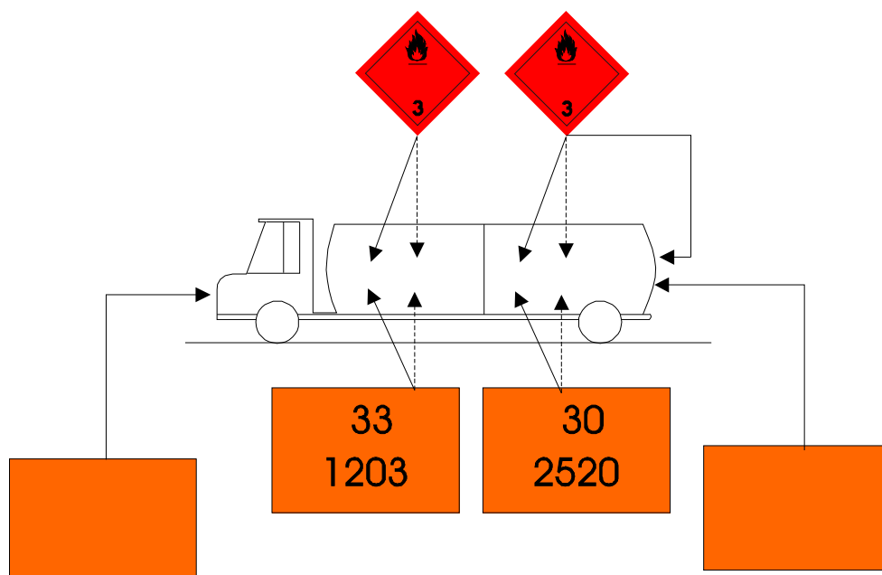
Fig. 2 Vehículo Cisterna cargado con dos o más Mercancías Peligrosas de la misma Clase o División (*)
