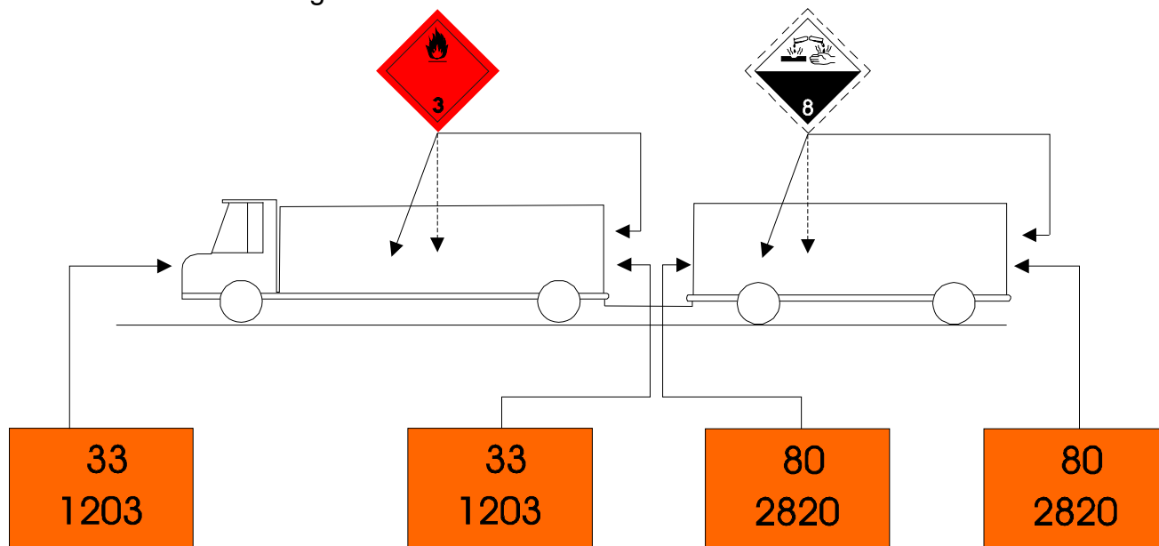
Fig. 7 Tren de Carretera cargado (Camión y Remolque) con dos o más Mercancías Peligrosas de Diferente Clase o División
